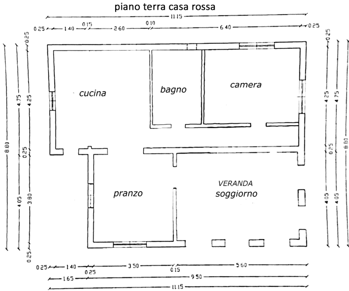
2 – Tenuta Feraxi Paradise - Casa Rossa – piano terra
