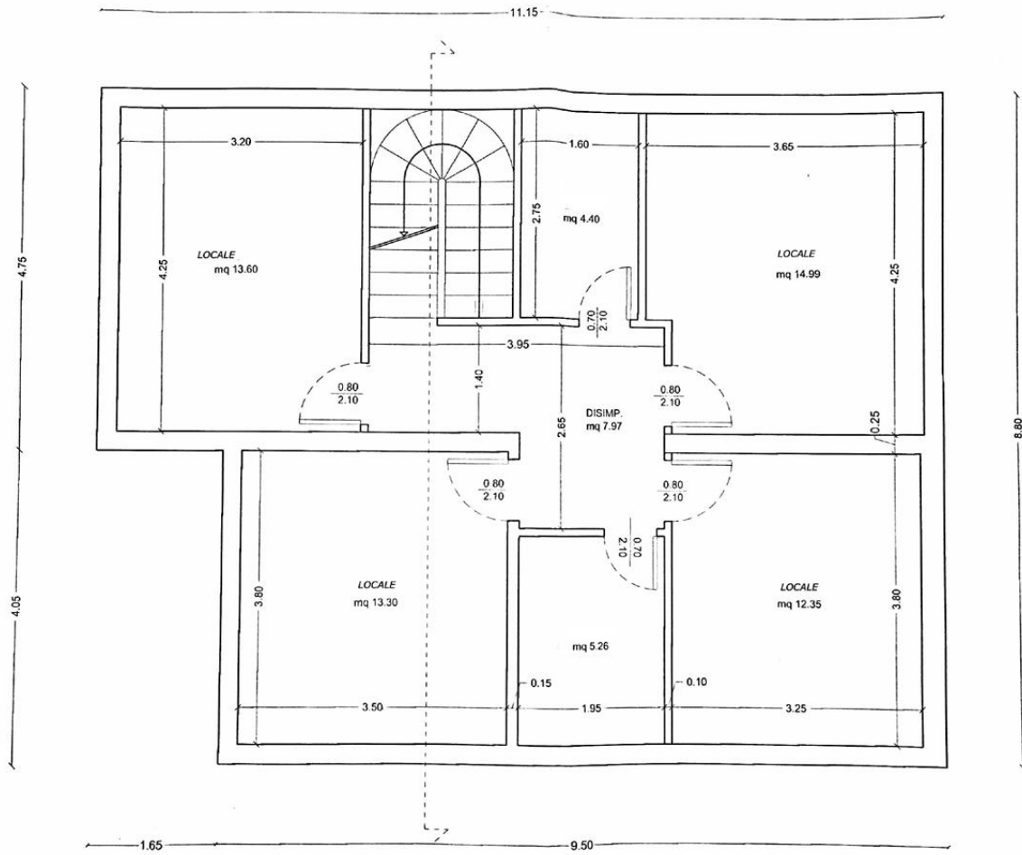
PIANTA PIANO PRIMO - STATO DI PROGETTO
