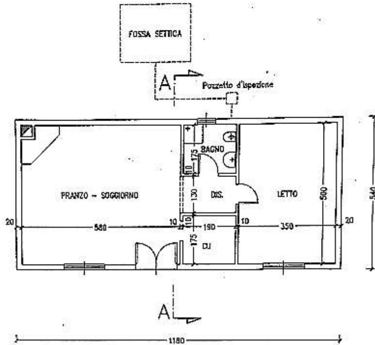
PIANTA QUOTATA
