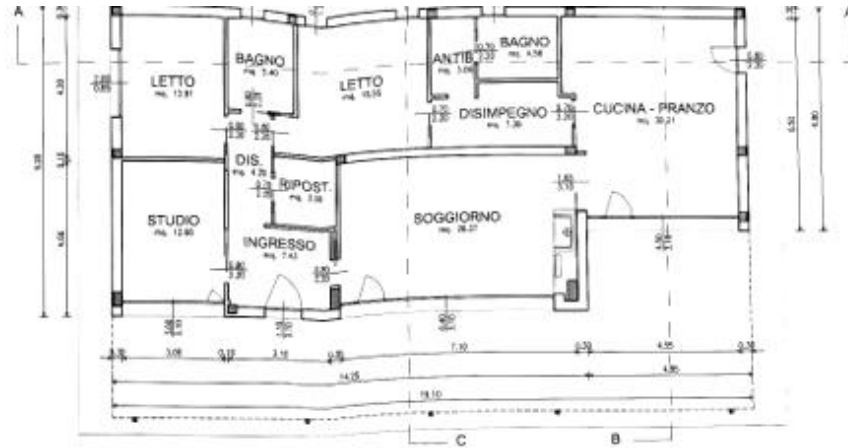
PIANTA QUOTATA
